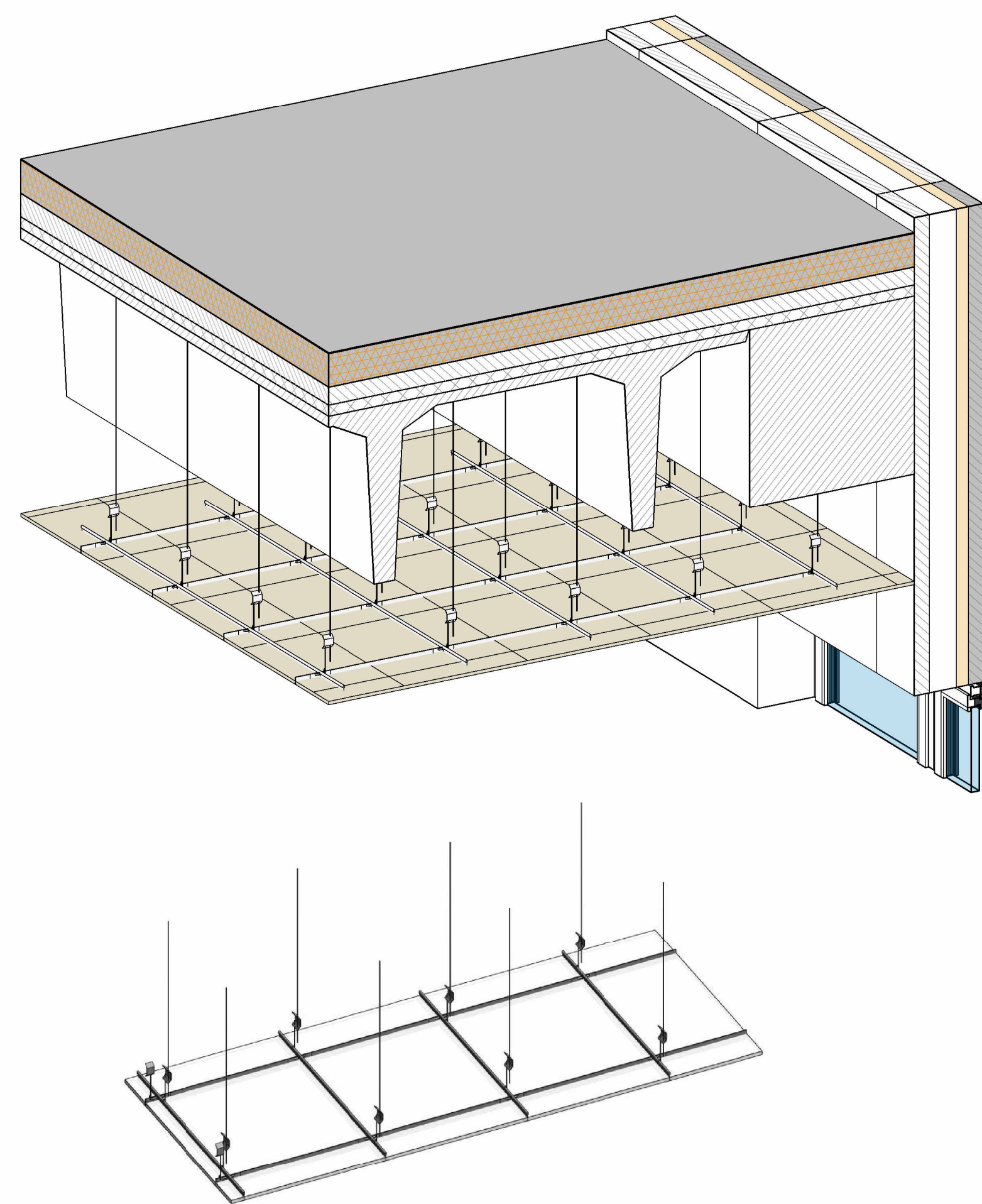
4 SCHEMA TIPOLOGICO DI POSA
