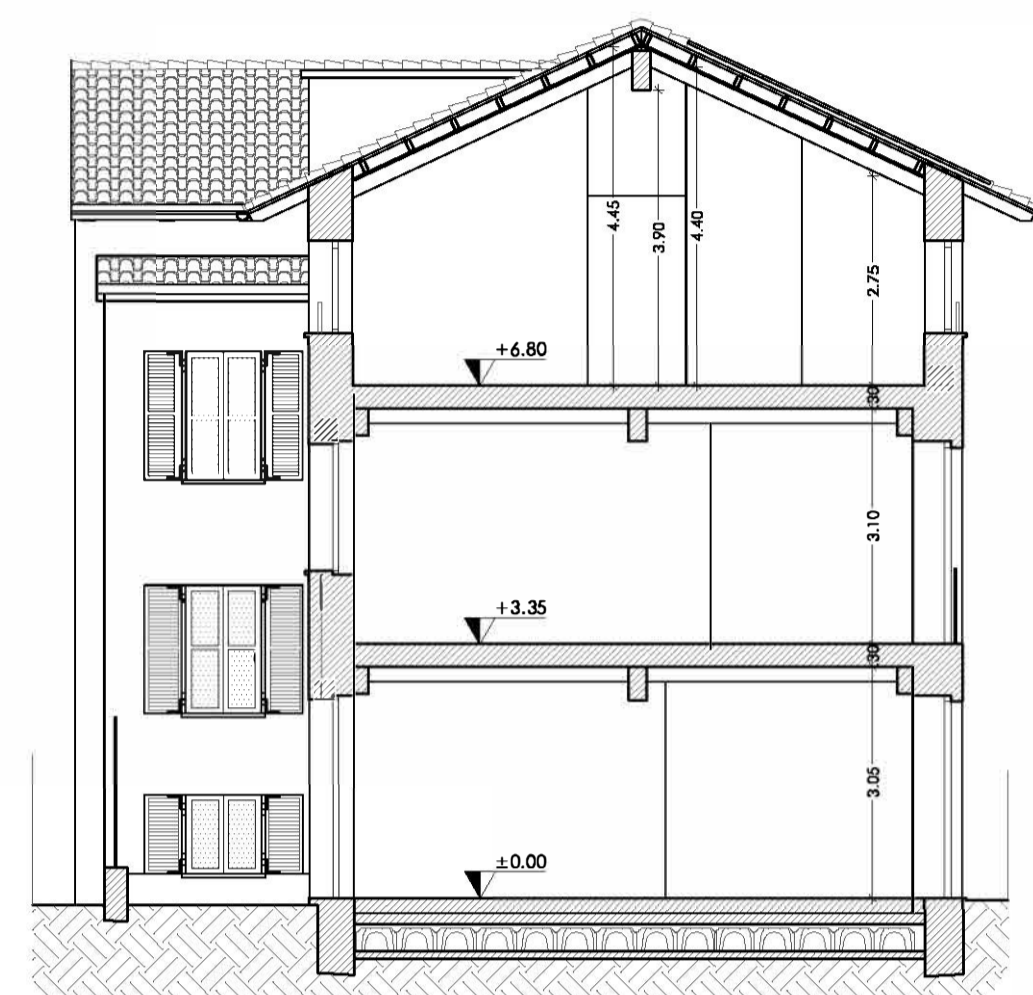
SEZIONE A.-A.
