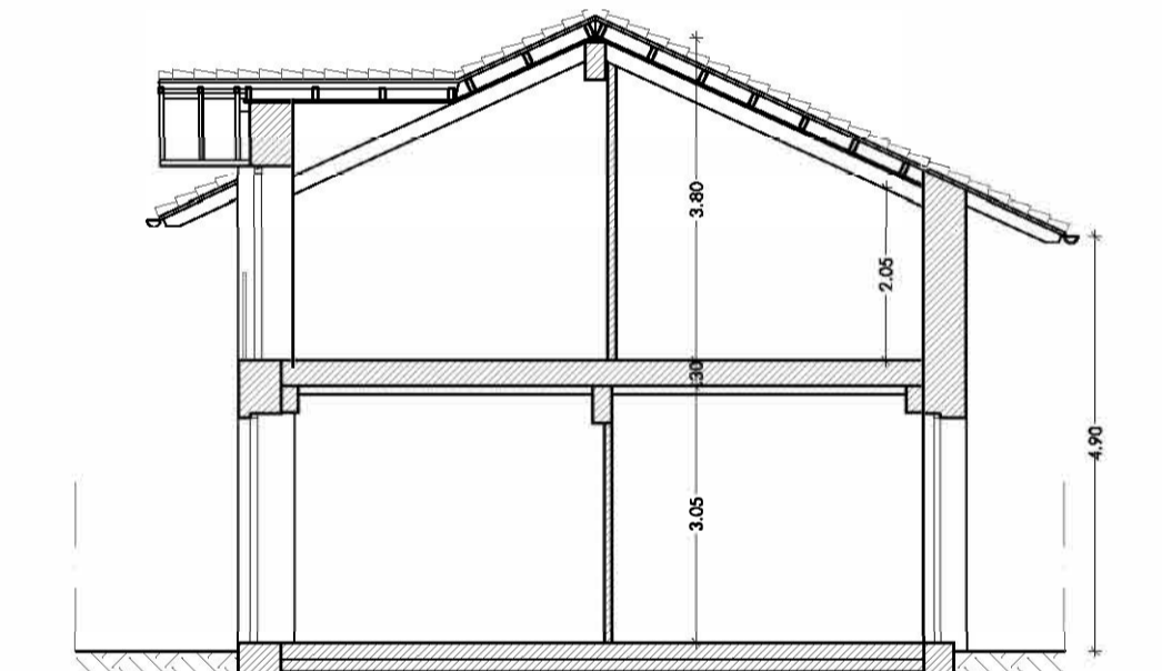
SEZIONE B.-B.
