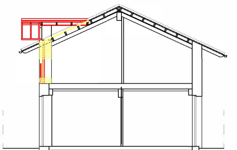
SEZIONE B.-B.
