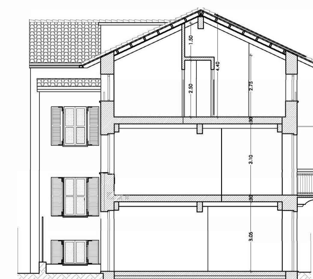
SEZIONE A.-A.
