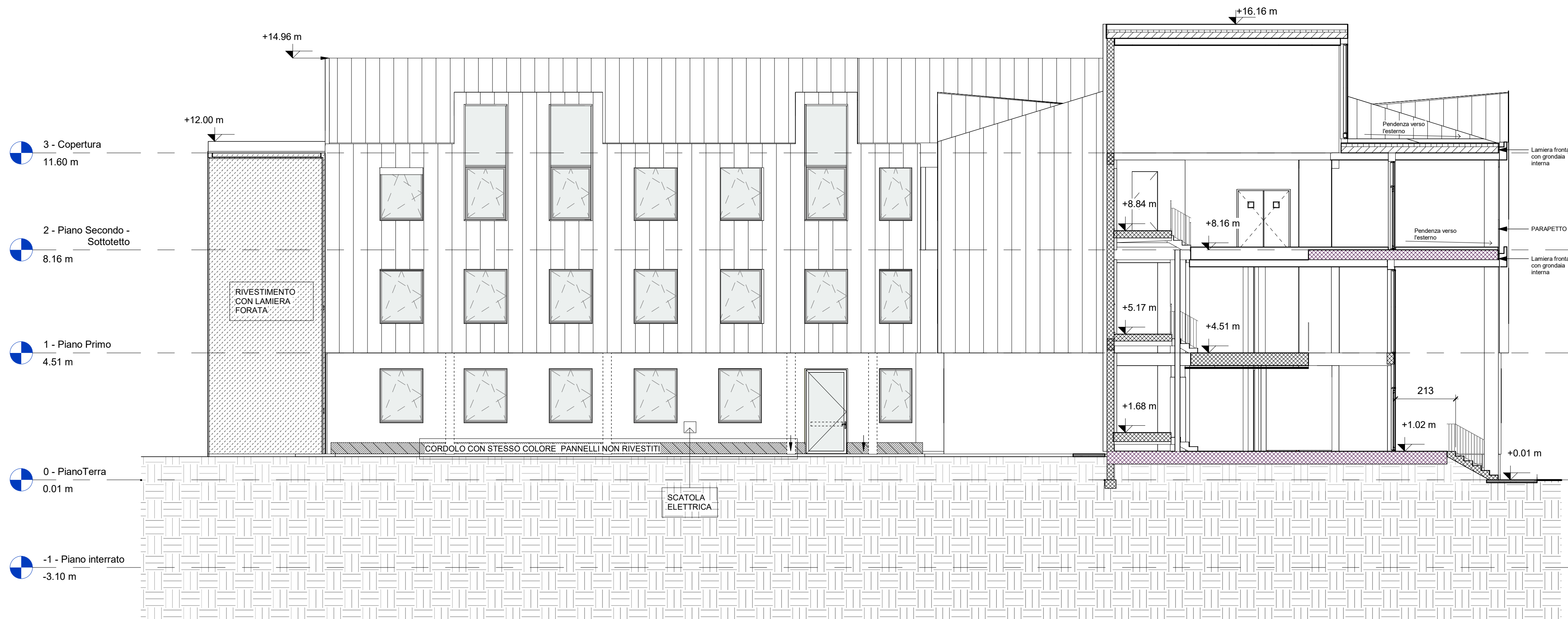
2 Facciata Sud, abaco moduli Copy 2 1 : 100
