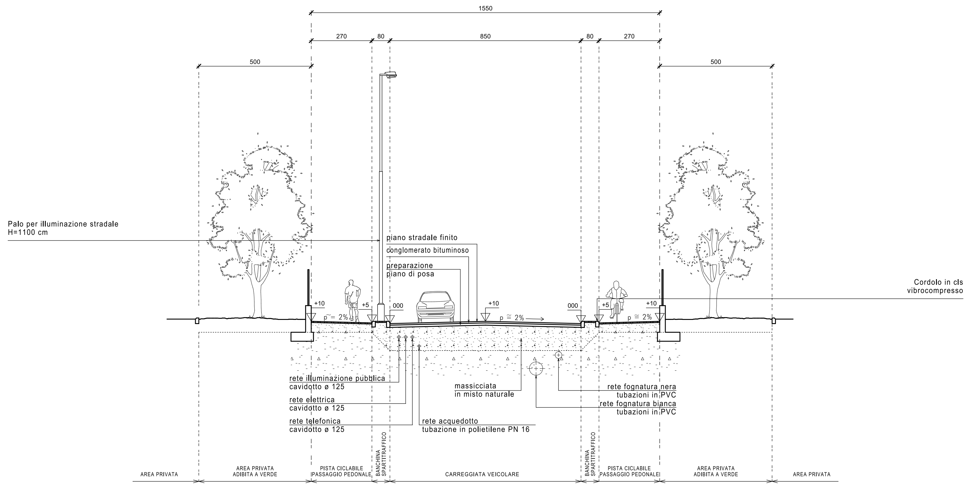
SEZIONE A-A - scala 1:100
