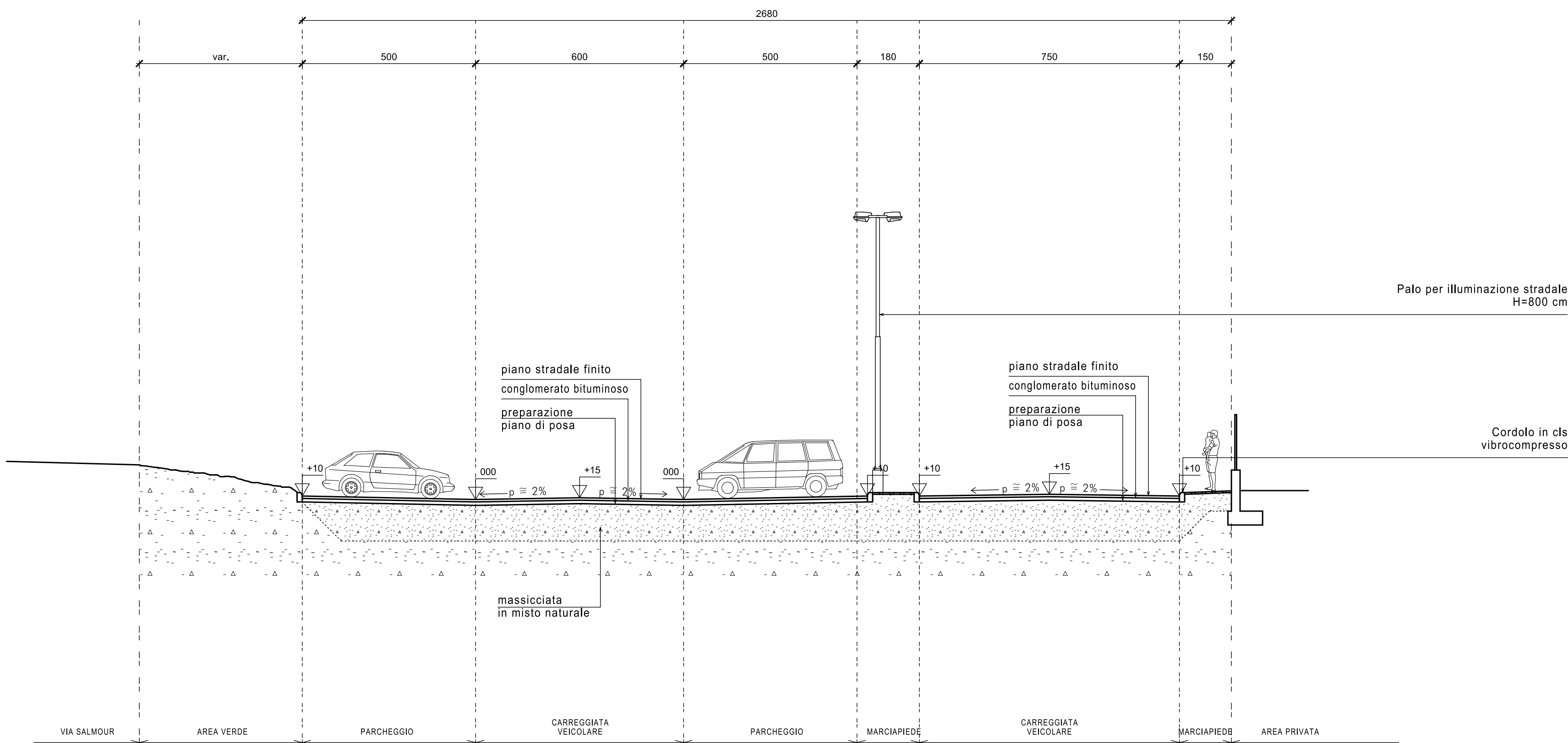
SEZIONE C-C - scala 1:100
