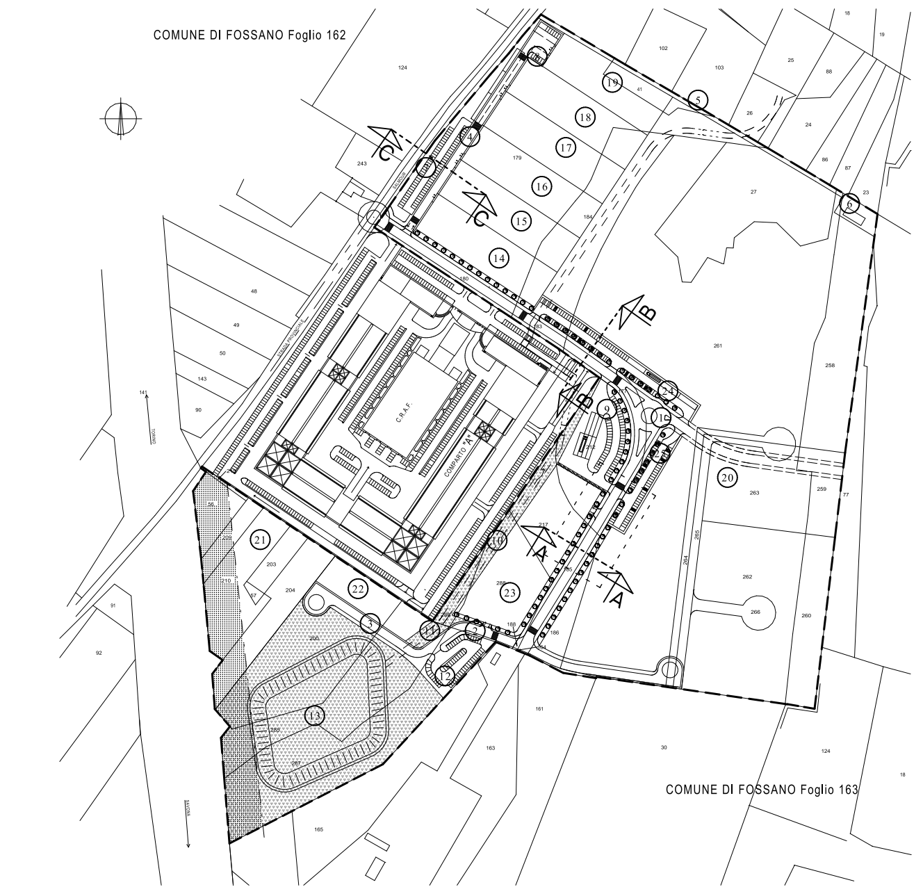
PLANIMETRIA - scala 1:5000
