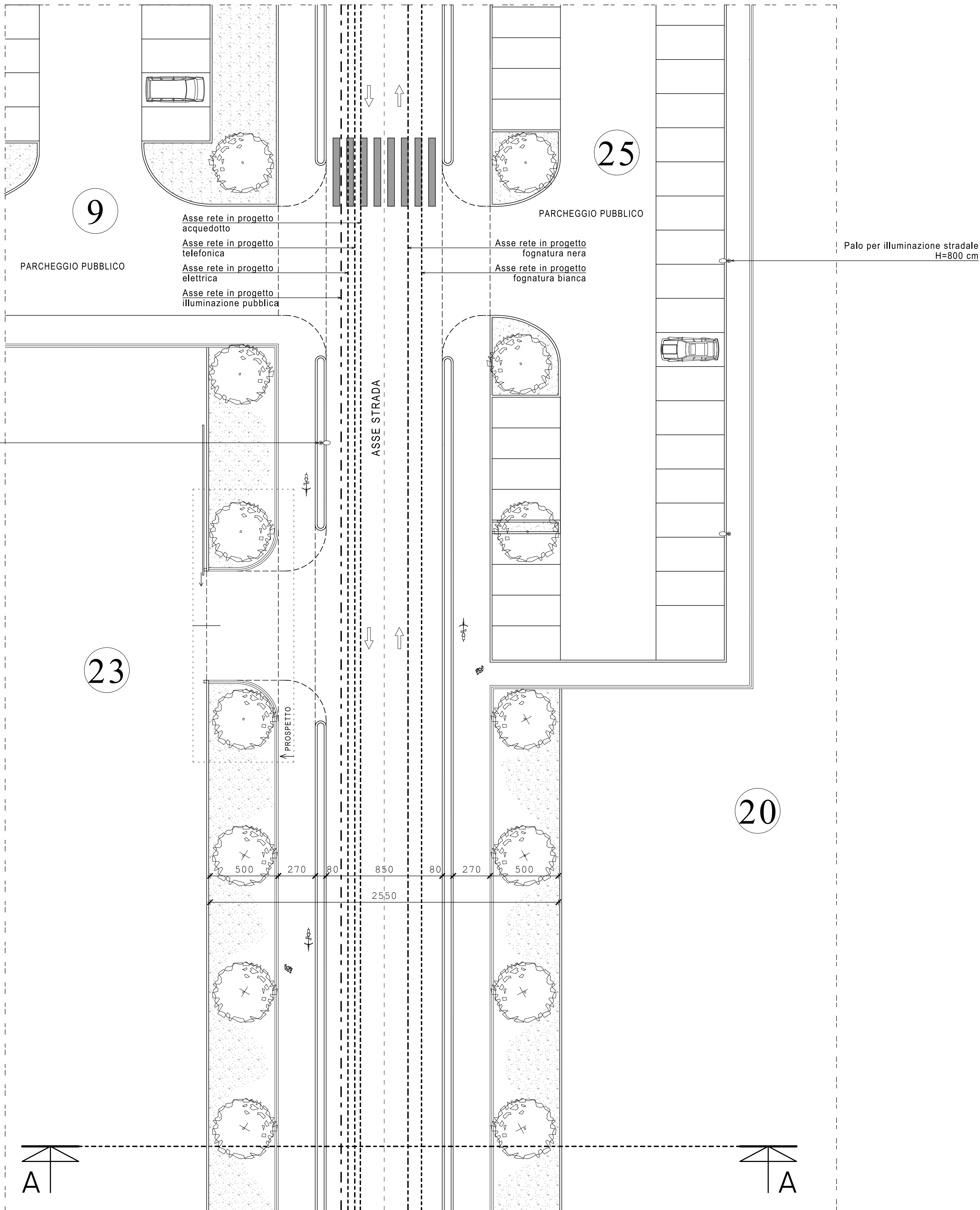
STRALCIO PLANIMETRICO - scala 1:200
