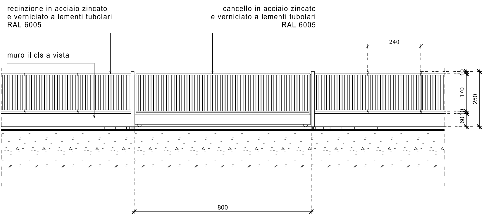
PROSPETTO - scala 1:100
