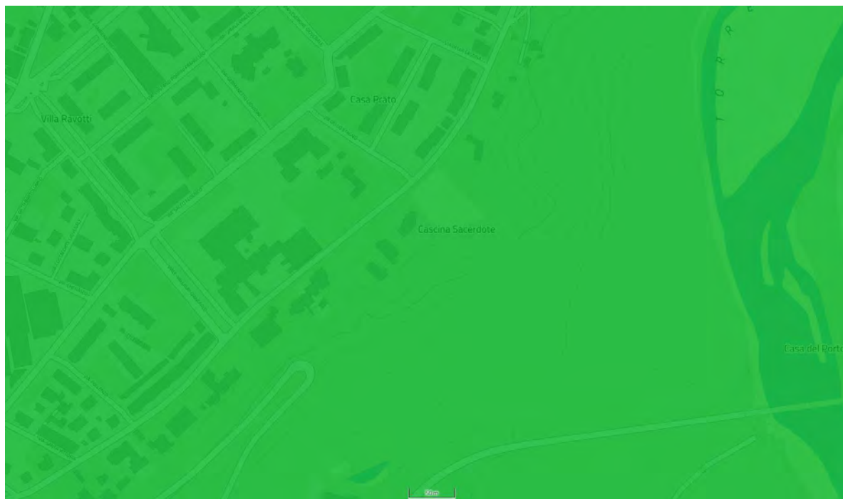
Figura 7 - AMBIENTE - Aree di superamento dei limiti della qualità dell'aria
