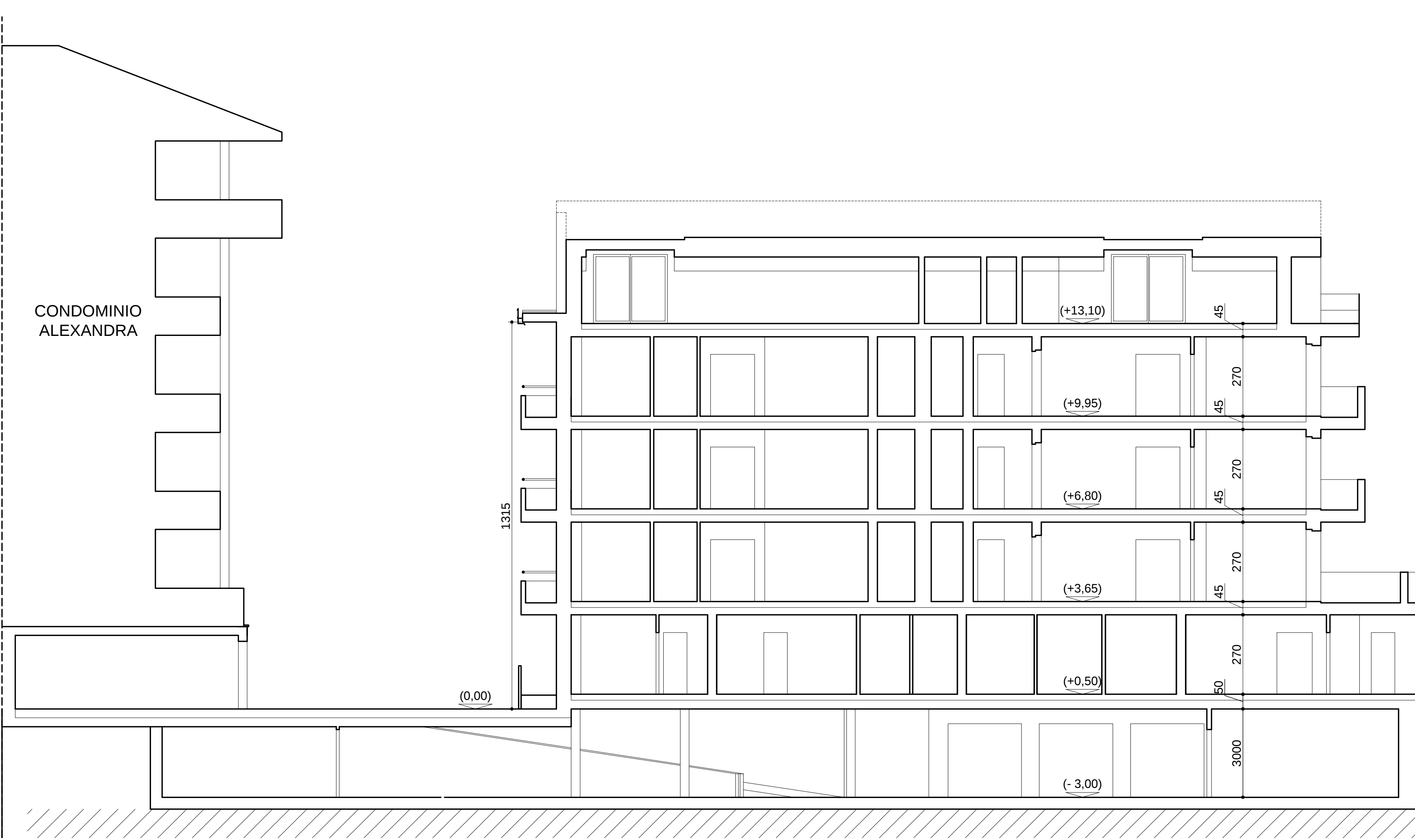
SEZIONE A - A'
