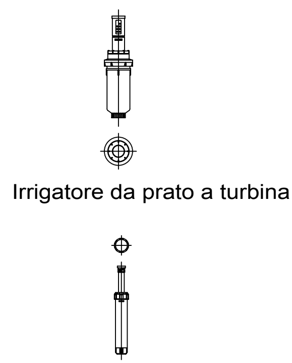
Irrigatore per giardino tipo "pop-up"
