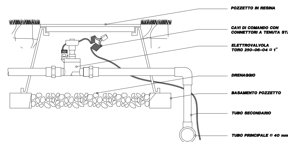
ELETTROVALVOLA Ø 1"
