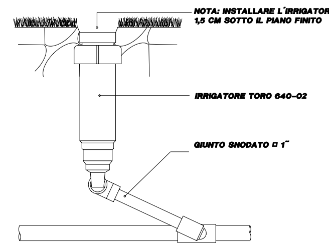
installazione IRRIGATORE
