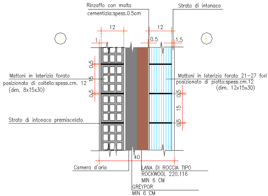
Figura 9 – muratura di tamponamento esterna
