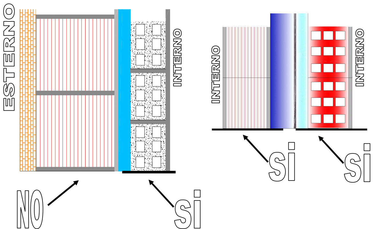
Figura 18 - Fascia tagliamuro ISOLMANT e/ostriscia sottoparete ISOLGOMMA ST 20 AD
