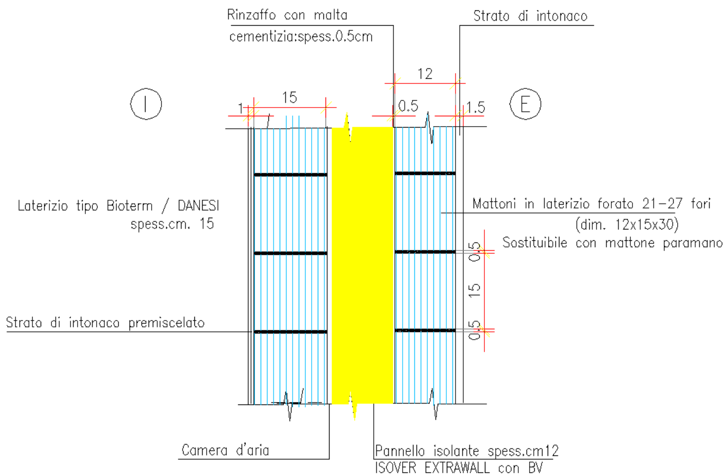
Figura 12 – muratura di tamponamento esterna
