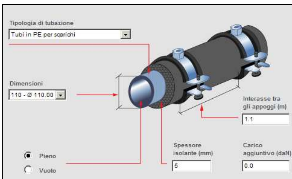
Figura 26 – modalità di posa del prodotto
