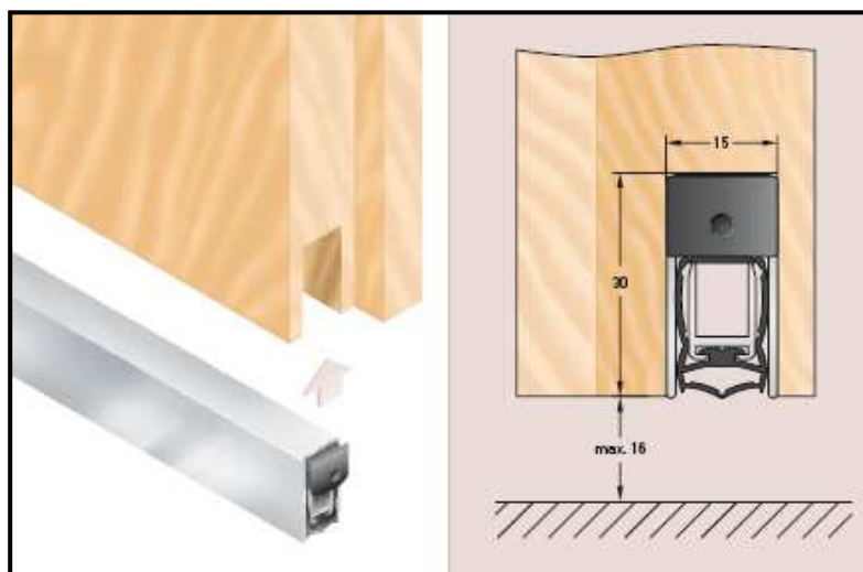
Figura 21 – guarnizione acustica per serramenti interni – antirumore/antifumo
