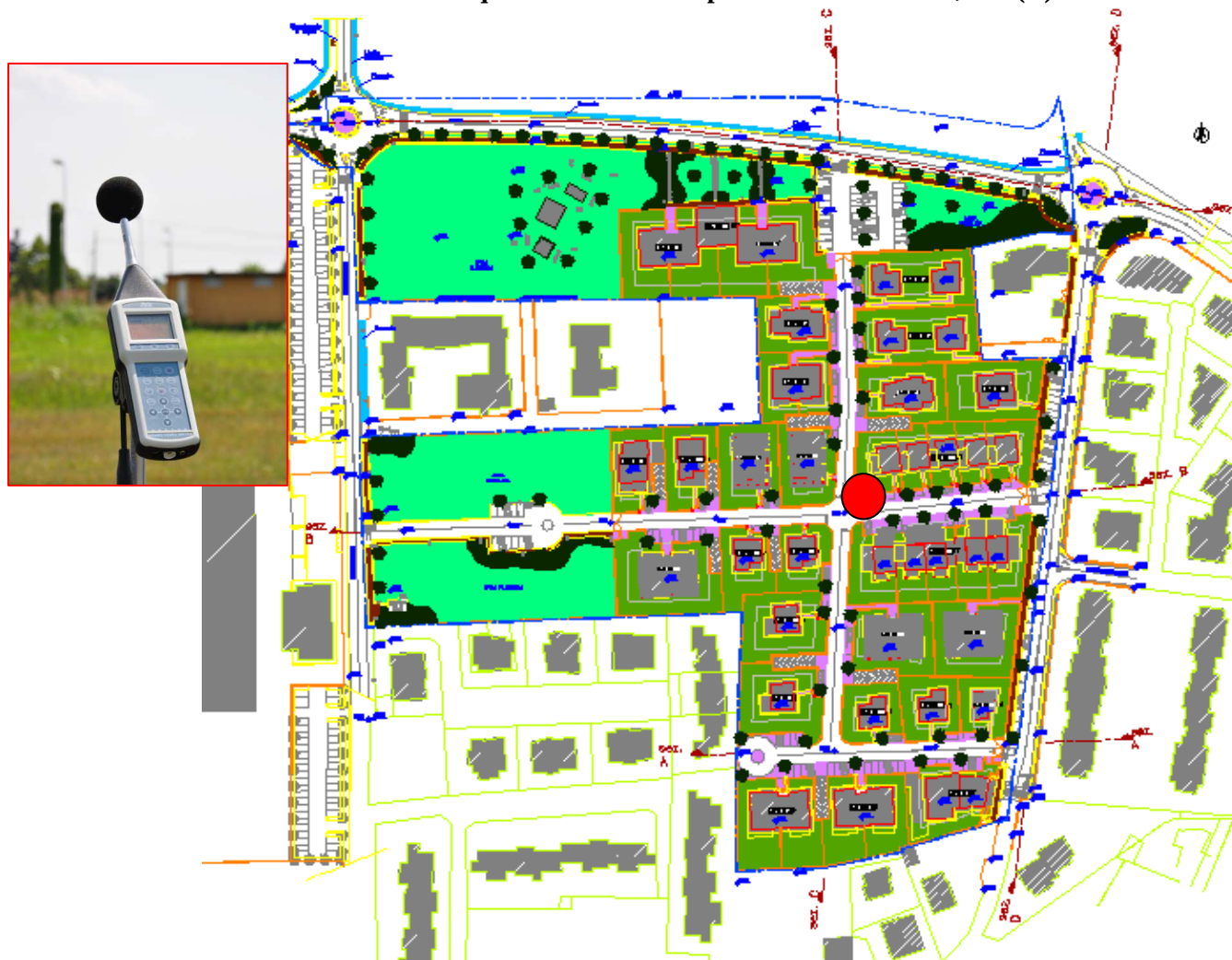
Figura 34 - punto di acquisizione fonometrica – centro pec
