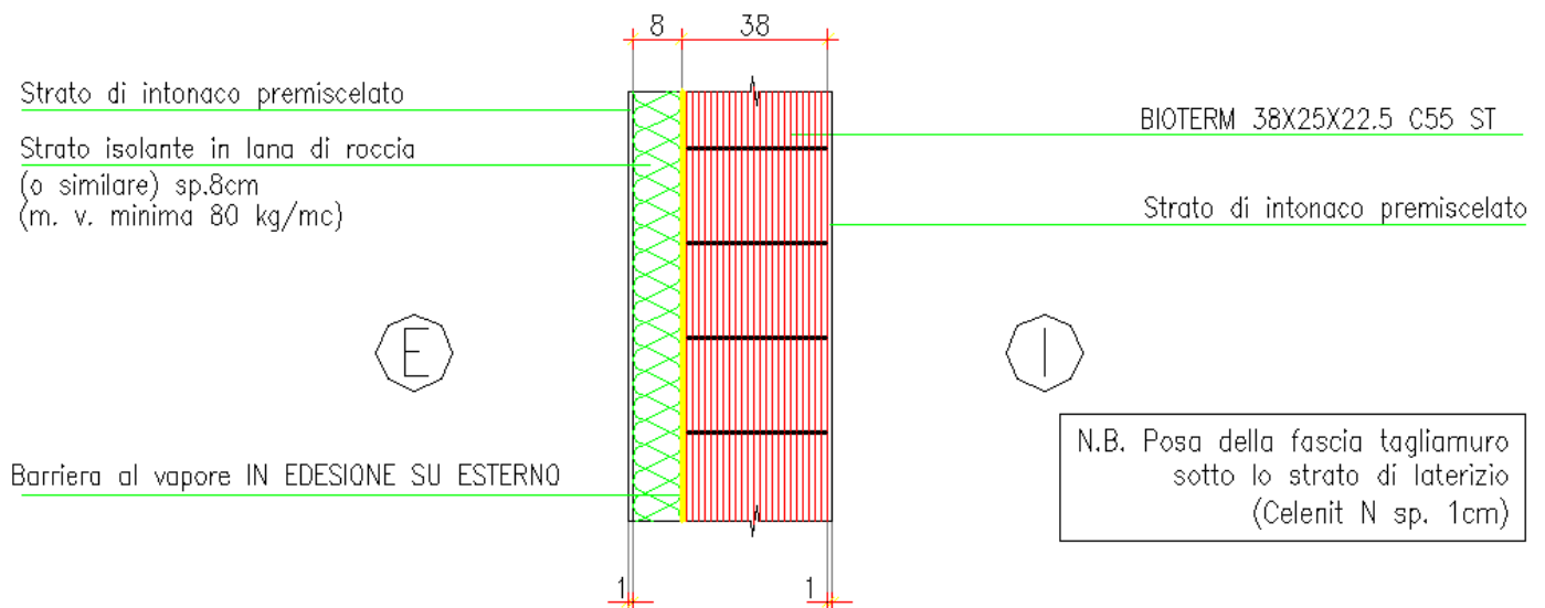
Figura 7 - Parete esterna
